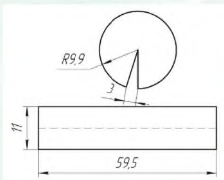
Тақияның сызбасы
