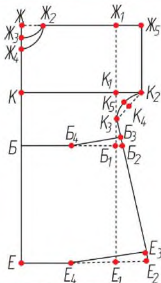
Жеңі тұтас пішілген иықты бұйымның сызбасы
