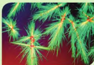
Тағамдық бояғыштардың кристалдары
