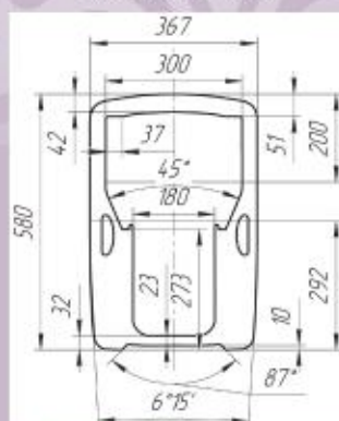
Олдинги тирагининг чизмаси
