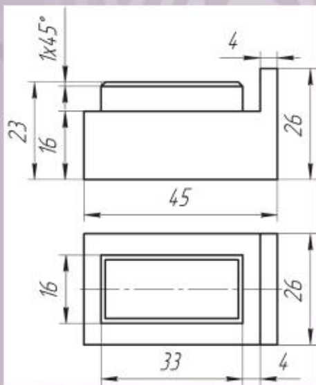
Деталь чизмаси (Тиқин. поз. номери 1)
