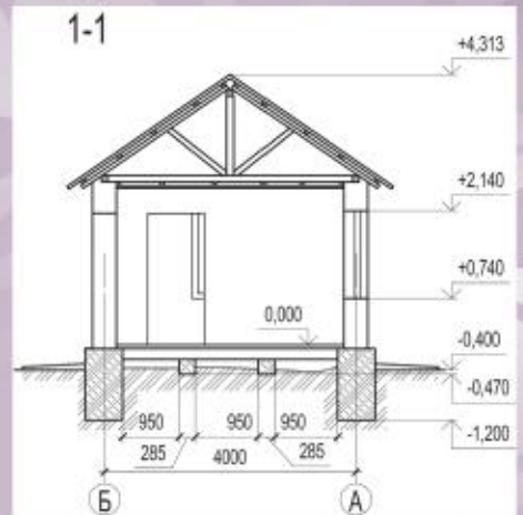
Кесим
