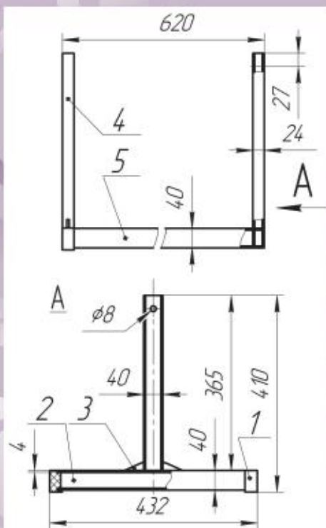
Умумий кўриниш чизмаси (Парта асосининг каркаси)
