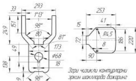
Суянчиғи ва ўриндиғининг чизмаси
