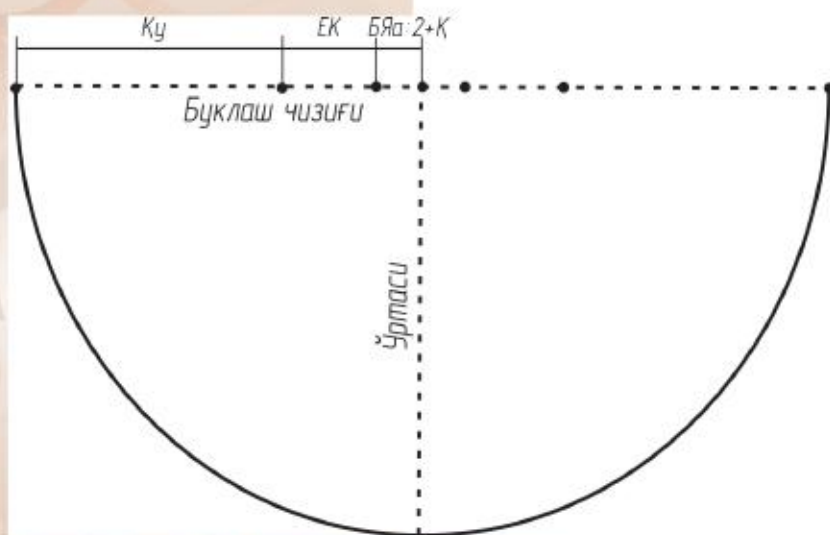
Пончо, туникани моделлаш
