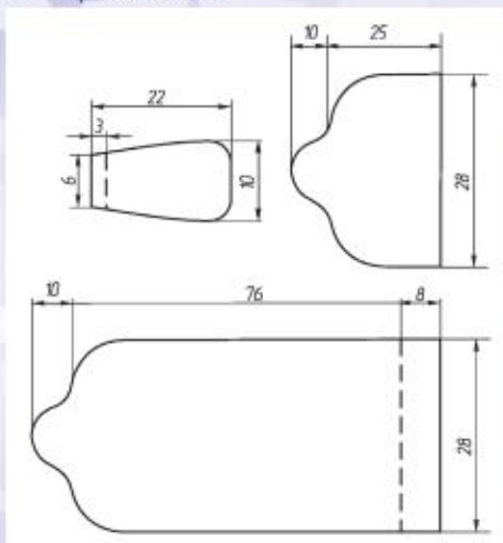
Буюмниң сизмиси
