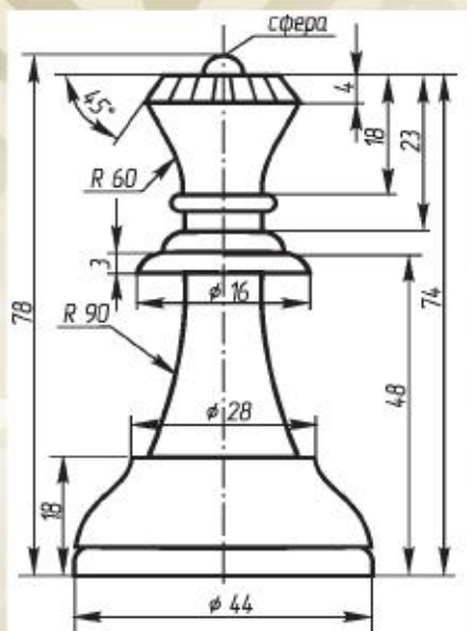
Чизма
