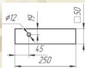
Асоснинг чизмаси
